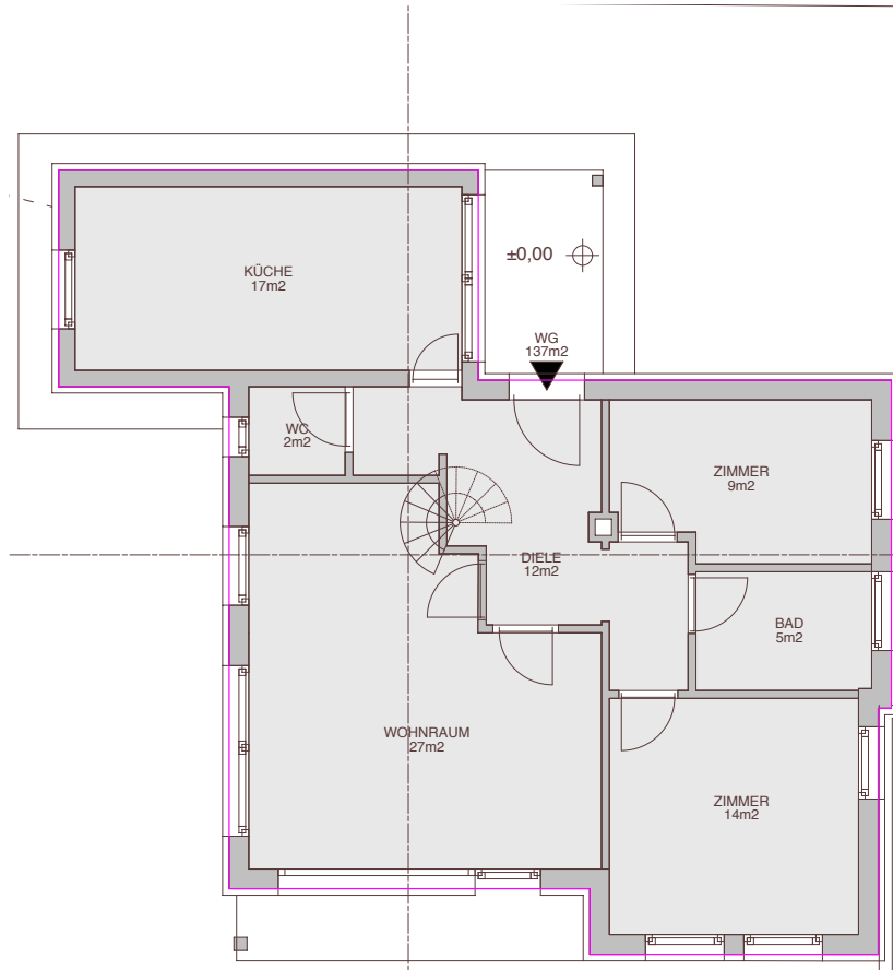
Untergeschoss
